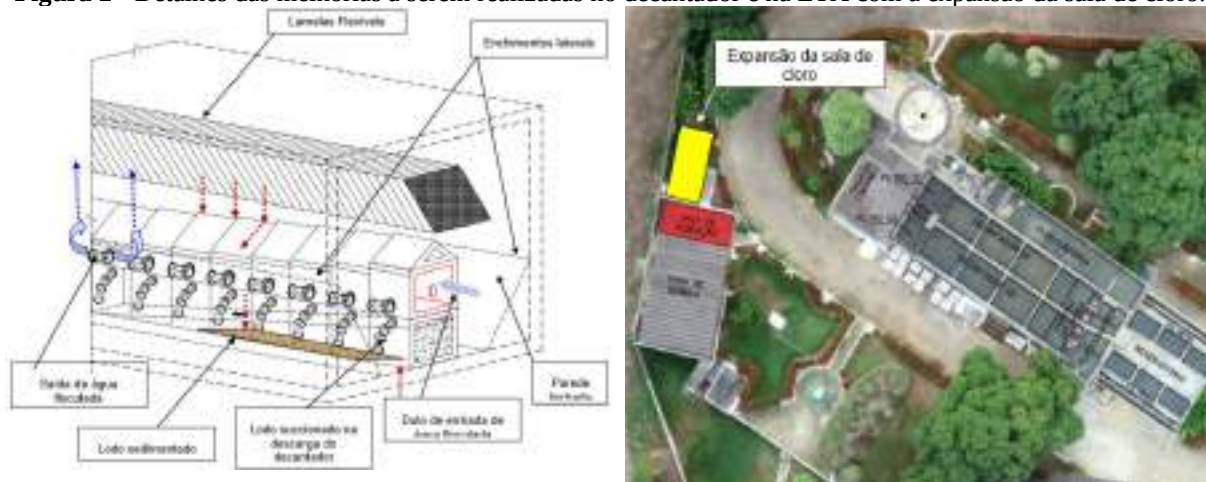
Figura 2 - Detalhes das melhorias a serem realizadas no decantador e na ETA com a expansão da sala de cloro.
